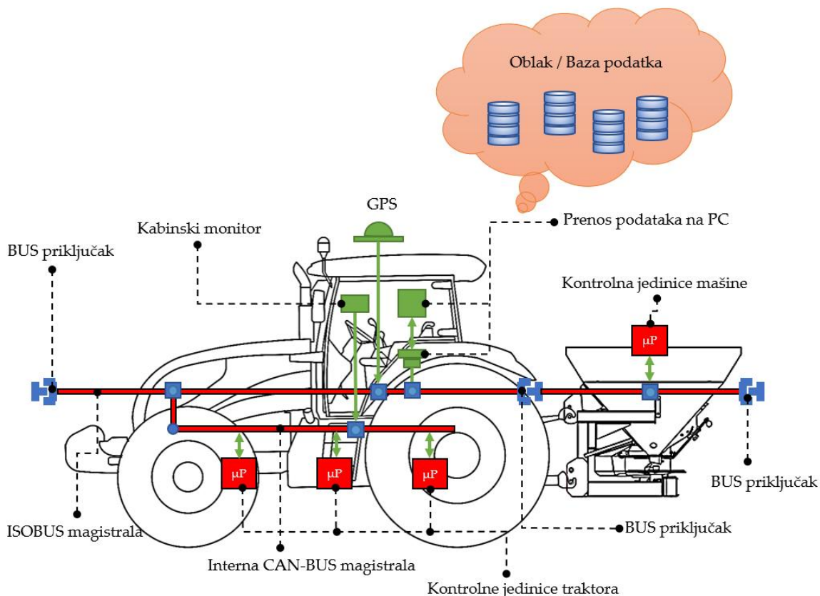
Slika 1.1. ISO-BUS komunikaciona šema
